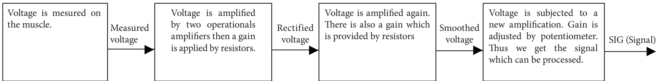
Fonctionnal diagram of Muscle Sensor v3
