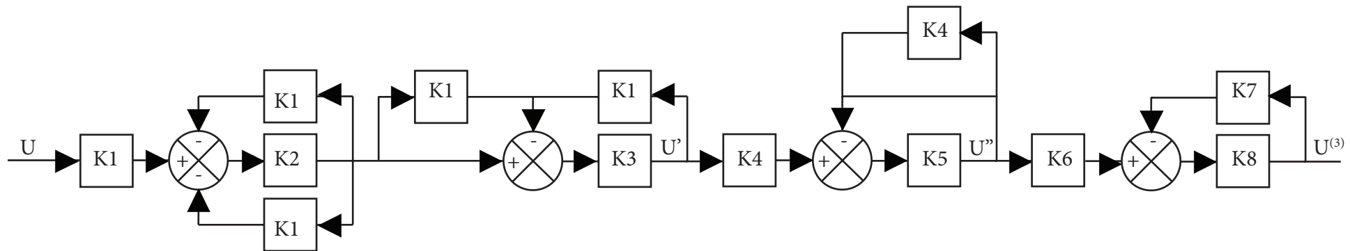
Schéma bloc Muscle Sensor v3
